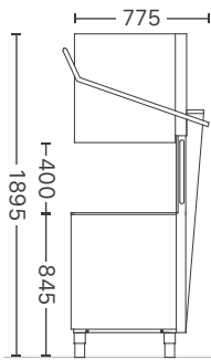
Fronte/Front
